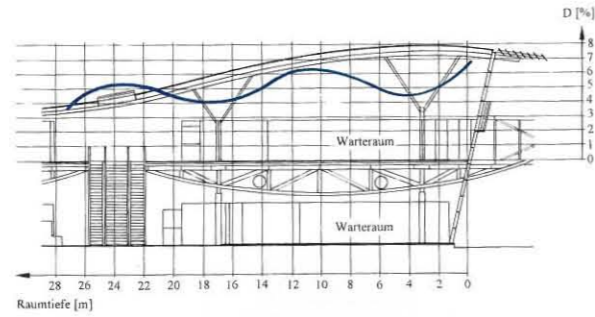
Tageslichtquotientenverlauf der aktuellen Planung Course of the day light-quotient of the new planning
